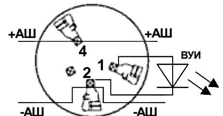
Рис. 1. Подключение базового основания В401L
