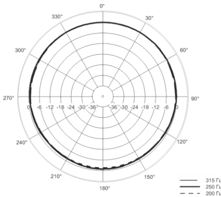
Диаграмма направленности в полярной системе координат в зависимости от частоты, Гц
