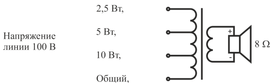
Рис. 2. Схема подключения оповещателя.
