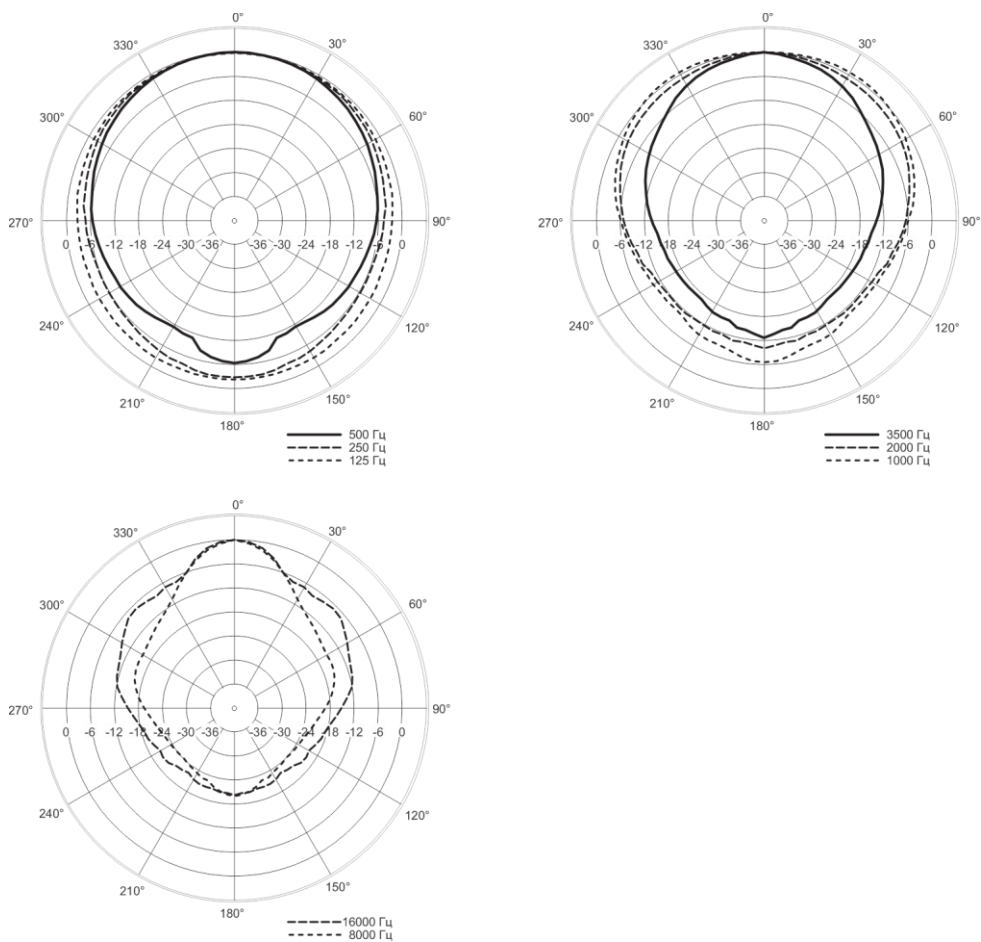
Диаграмма направленности в полярной системе координат в зависимости от частоты, Гц
