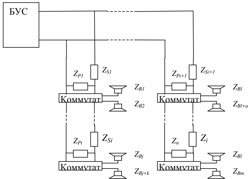
Рисунок 6.9. Схема измерения импеданса линий оповещения.
