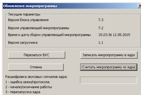
Рисунок 7.56. Диалоговое окно обновления микропрограммы главного микроконтроллера БУС.
