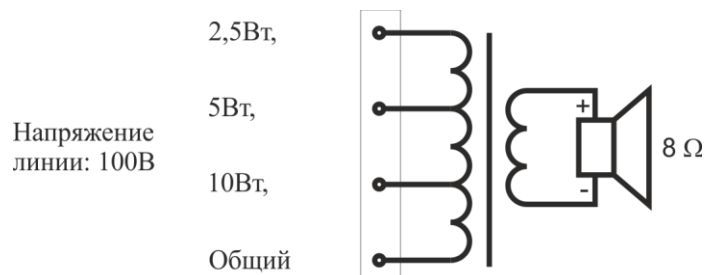
Рис. 2. Схема подключения оповещателя.
