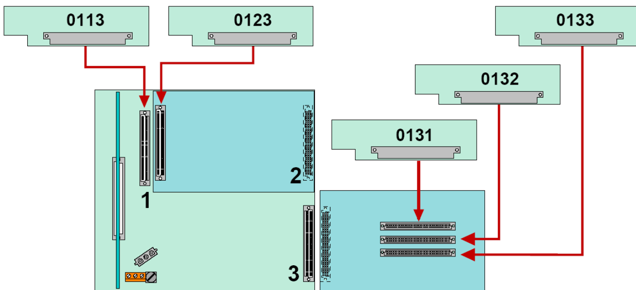
Рис. 44: Пример: КП пожарной сигнализации IQ8Control
