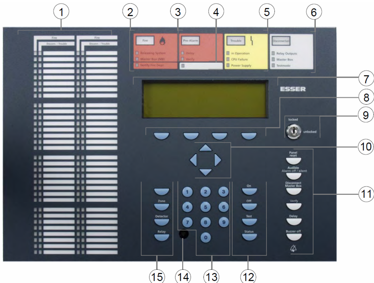
Рим. 1: Обзор элементов индикации и управления
