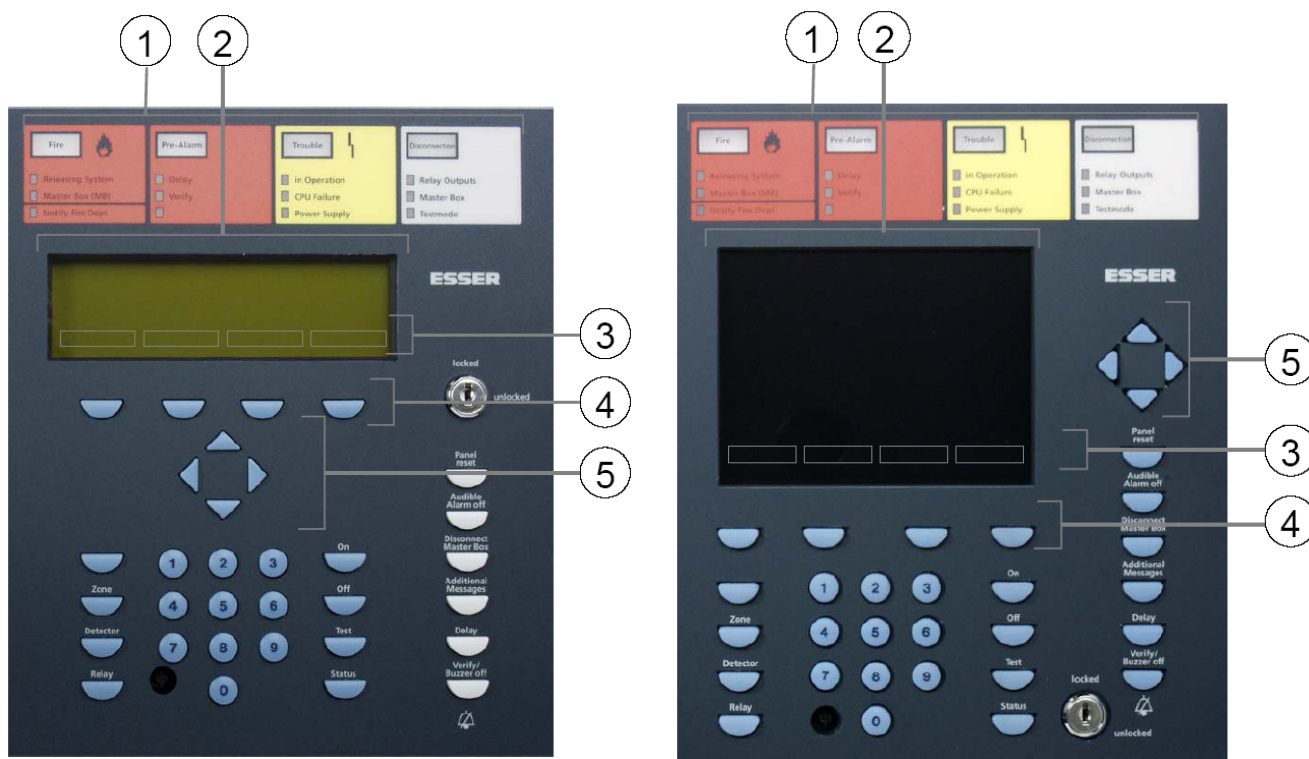
Рис. 4: Пульт управления – Клавиатура – Стандартный дисплей Пульт управления – Клавиатура – Дисплей 1/4-VGA
