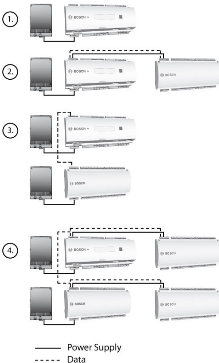
Рис. 4.8: Примеры конфигураций
