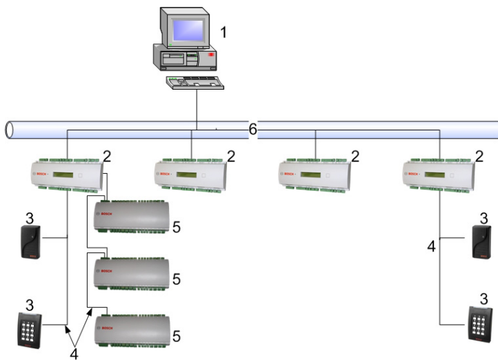
Рис. 3.6: Обзор системы
