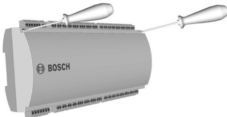
Рис. 4.3: Открывание корпуса AMC2-16IOE
