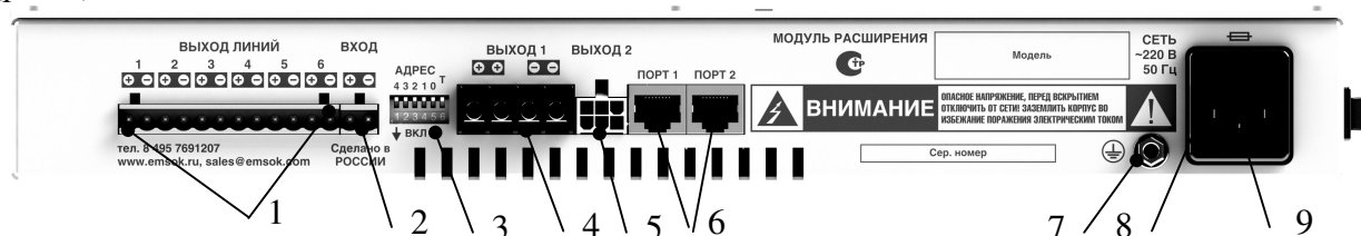
Рис. 2. Нижняя панель модуля расширения. 1 – выход линий (коммутируемый), 2 – резервный вход коммутатора, 3 – переключатель адреса, 4, 5 – некоммутируемые выходы модуля расширения, 6 – порт связи, 7 – клемма защитного заземления, 8 – сетевой предохранитель, 9 – соединитель сетевого питания.
