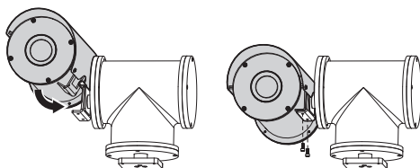
Рис. 07 Поворотное устройство.
