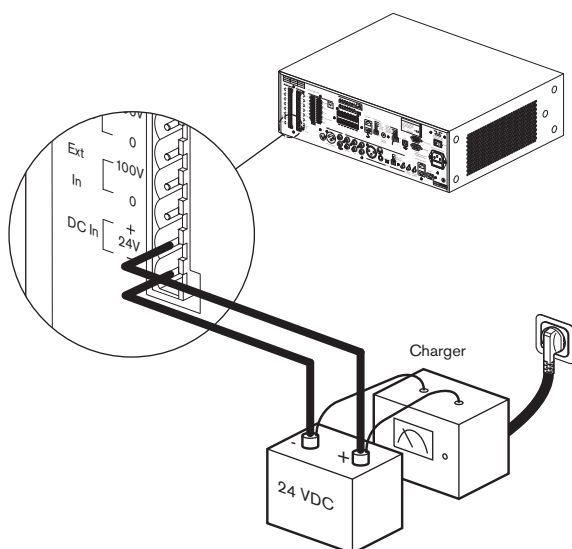
Рисунок 5.18: Подключение резервного источника питания
