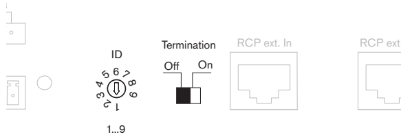
Рисунок 6.9: Настройки панели удаленного управления
