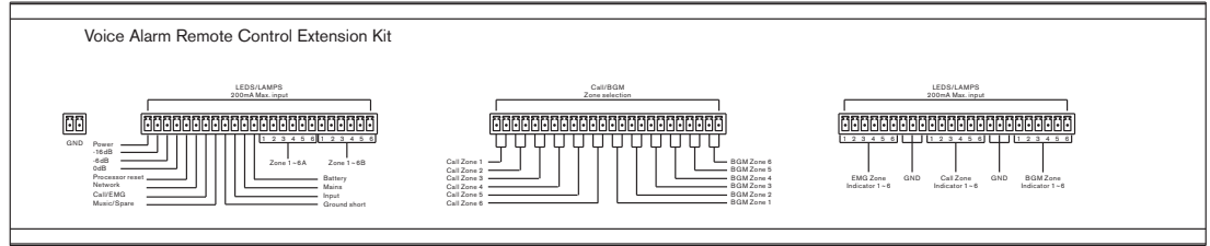
Рисунок 3.12: Вид набора расширителя панели удаленного управления спереди и сзади
