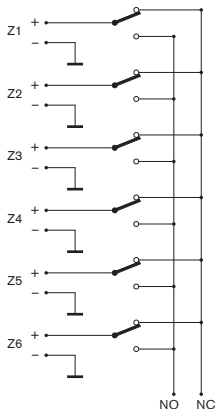
Рисунок 5.8: Контакты выхода обхода регулятора громкости
