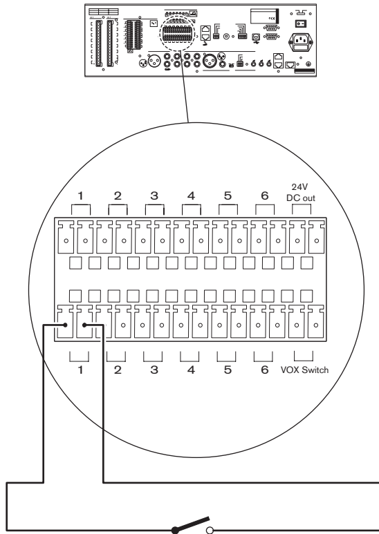
Рисунок 5.20: Подключение служебных триггерных входов
