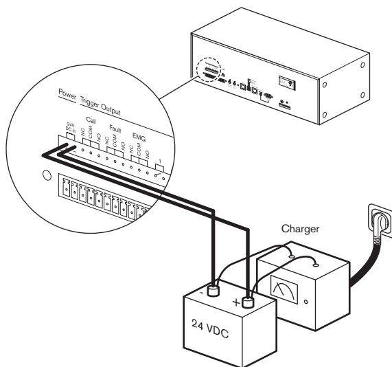
Рисунок 5.29: Подсоединение источника электропитания
