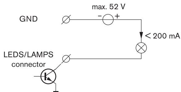
Рисунок 5.27: Подключение ламп
