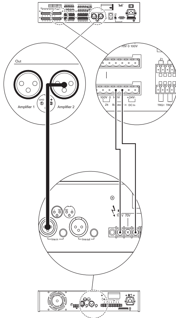
Рисунок 5.22: Подключение внешнего усилителя мощности 2
