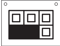
Рисунок 4.3: JP1 для одной платы контроля линии
