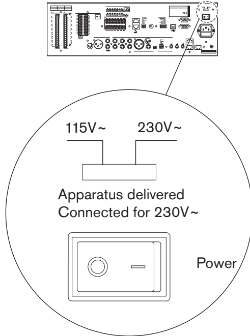
Рисунок 5.16: Селектор напряжения
