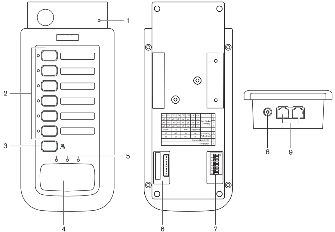
Рисунок 3.7: Виды вызывной станции сверху и снизу
