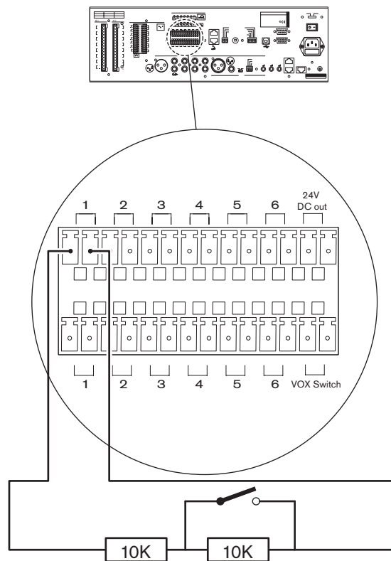
Рисунок 5.19: Подключение тревожных триггерных входов
