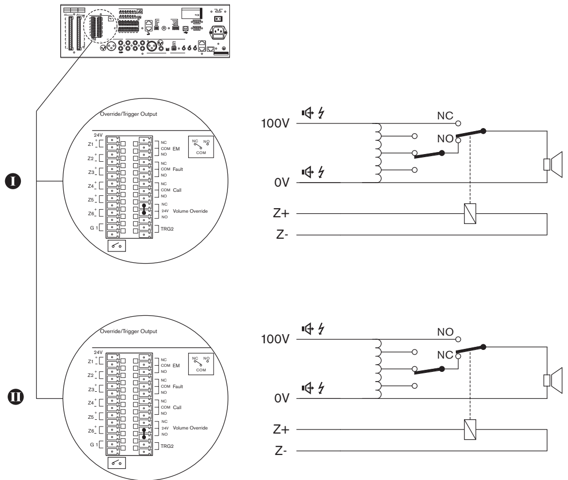
Рисунок 5.9: 4-проводная схема подключения регуляторов громкости
