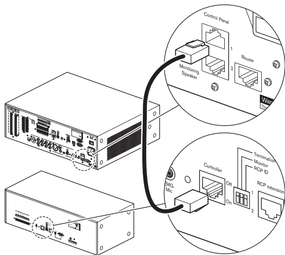
Рисунок 5.5: Подключение панели удаленного управления
