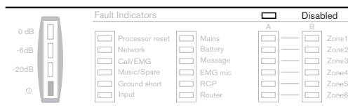
Рисунок 6.2: Индикатор "Disabled" (Отключено)
