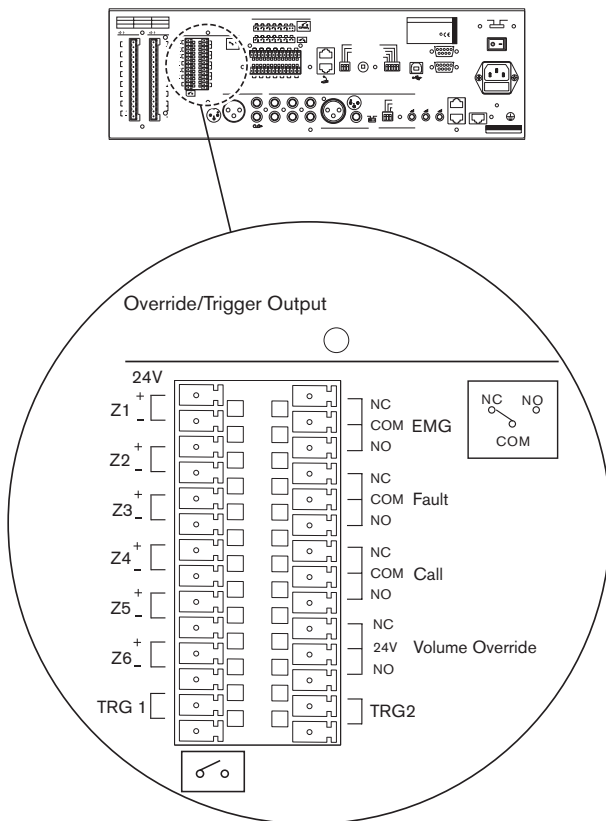
Рисунок 5.7: Выходы обхода регуляторов громкости
