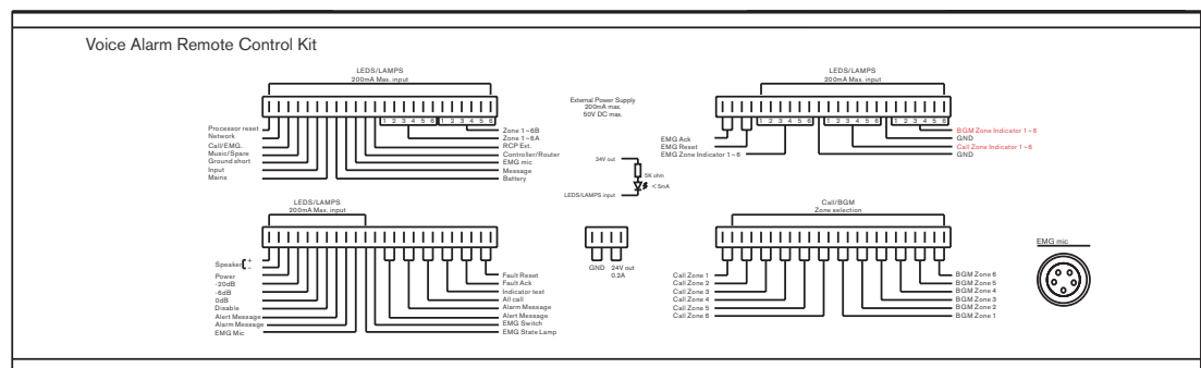
Рисунок 3.10: Вид набора для панели удаленного управления спереди и сзади
