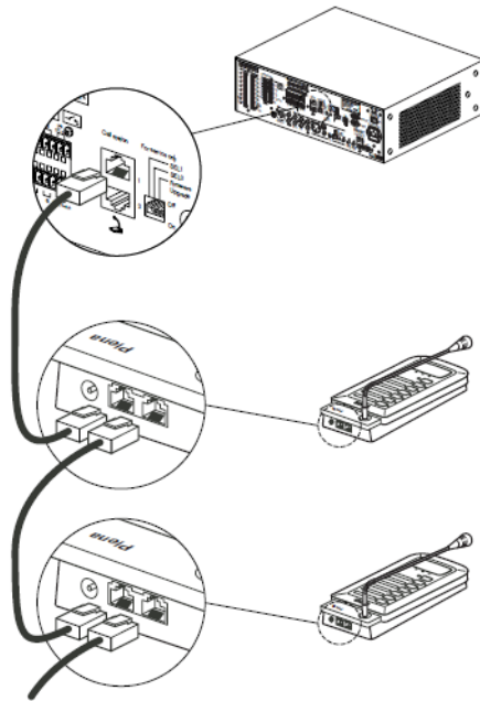
Рисунок 5.2: Подключение вызывных станций
