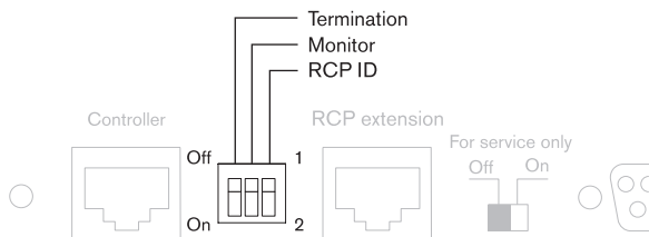
Рисунок 6.8: Настройки панели удаленного управления
