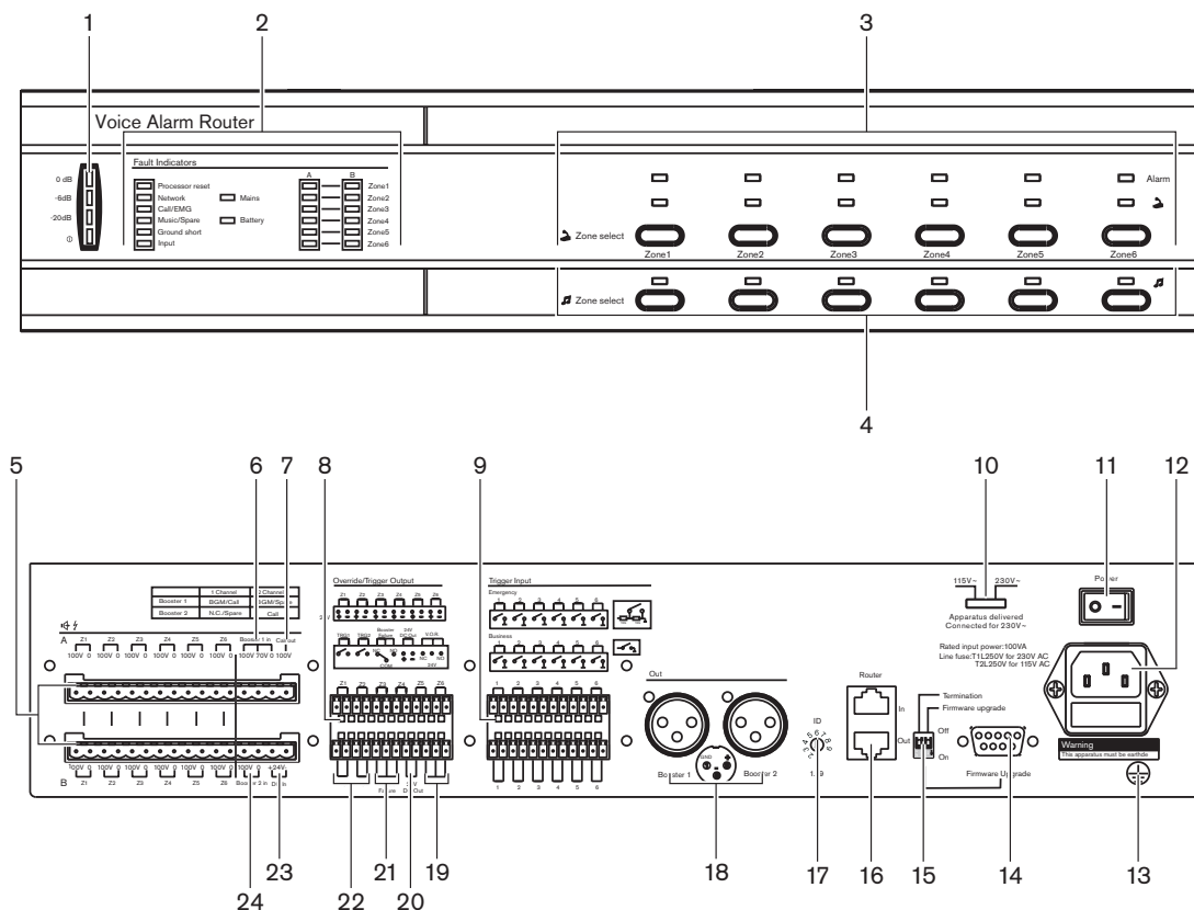
Рисунок 3.4: Вид маршрутизатора системы оповещения спереди и сзади
