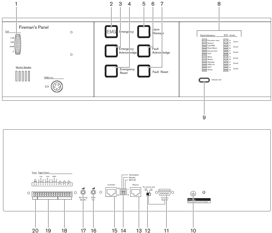
Рисунок 3.13: Вид панели пожарного спереди и сзади
