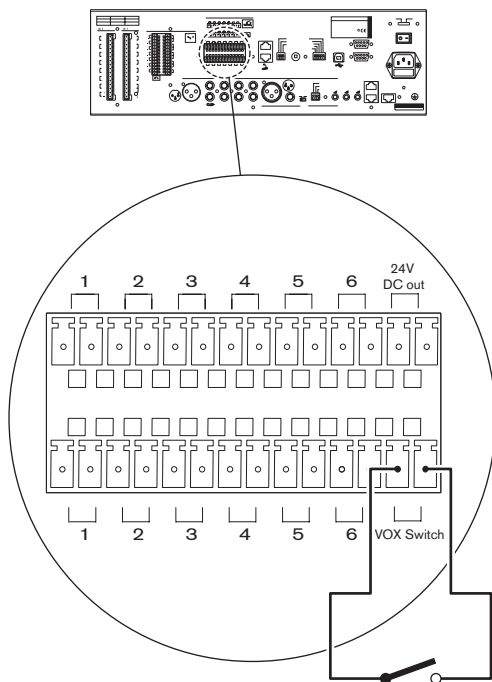
Рисунок 5.13: Подключение переключателя VOX
