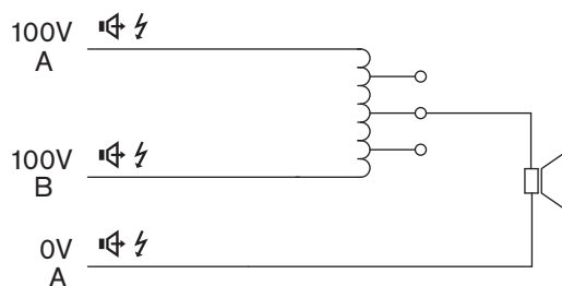
Рисунок 5.10: 3-проводная схема подключения регуляторов громкости
