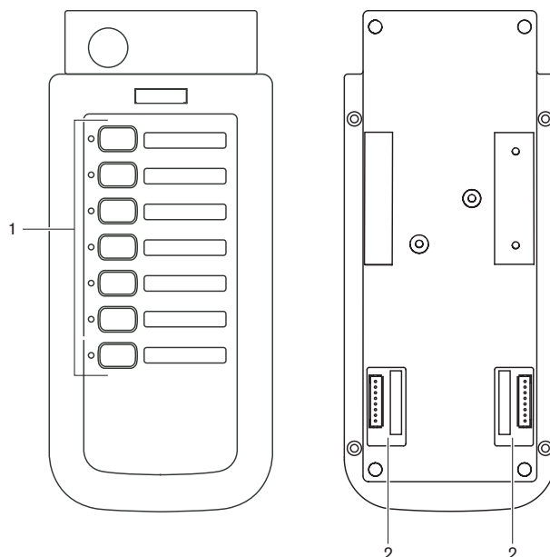
Рисунок 3.8: Виды клавиатуры вызывной станции сверху и снизу
