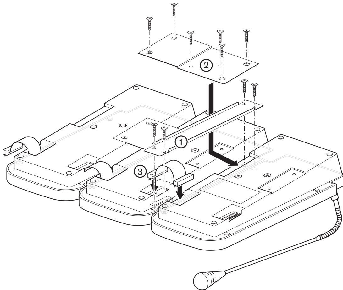
Рисунок 4.2: Подключение клавиатур вызывной станции
