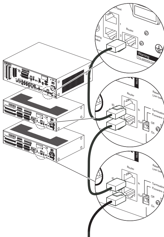
Рисунок 5.3: Подключение маршрутизаторов
