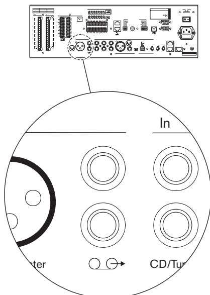
Рисунок 5.11: Линейный выход
