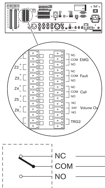
Рисунок 5.15: Контакты выхода состояния (по умолчанию)
