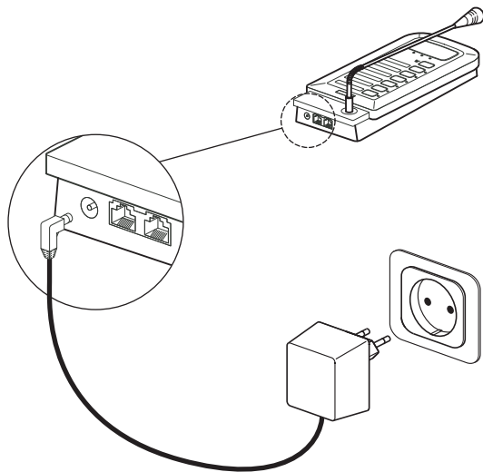
Рисунок 5.23: Подсоединение источника электропитания
