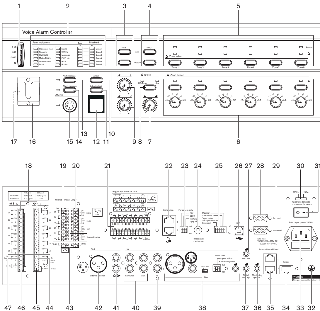
Рисунок 3.2: Вид контроллера системы оповещения спереди и сзади
