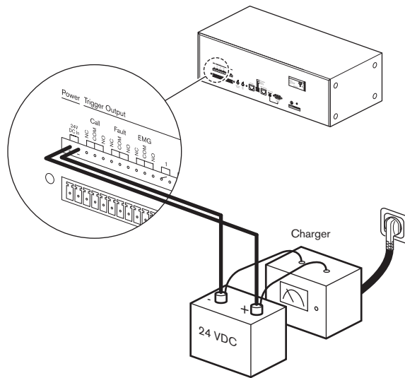
Рисунок 5.25: Подключение источника питания 24 В пост. тока
