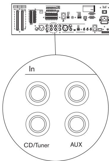
Рисунок 5.14: Входы фоновой музыки
