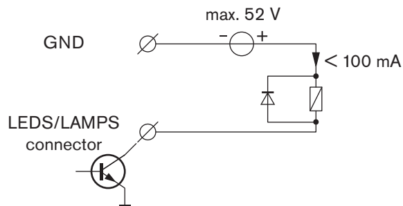
Рисунок 5.28: Подключение реле
