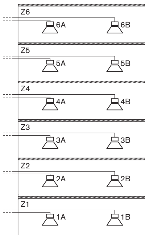
Рисунок 5.6: Подключение зон громкоговорителей
