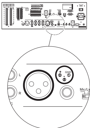
Рисунок 5.12: Вход "Mic/line" с функцией VOX
