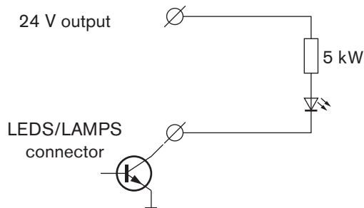
Рисунок 5.26: Подключение индикаторов
