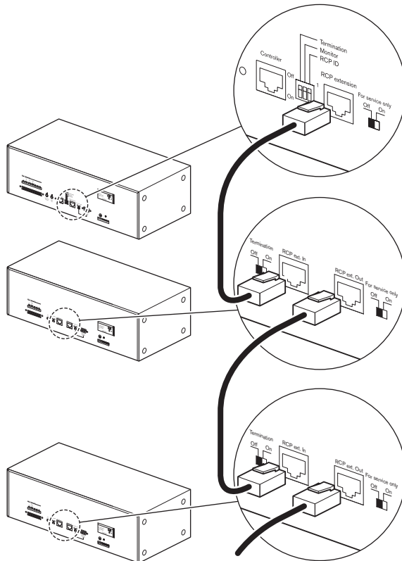
Рисунок 5.24: Подключение расширителей панели удаленного управления
