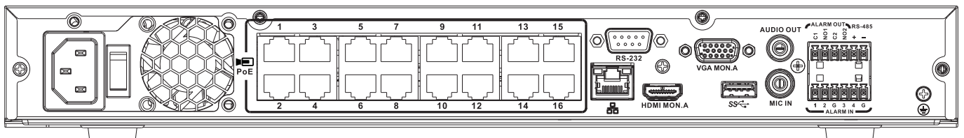
Задняя панель DIVAR network 2000 (16 PoE)
